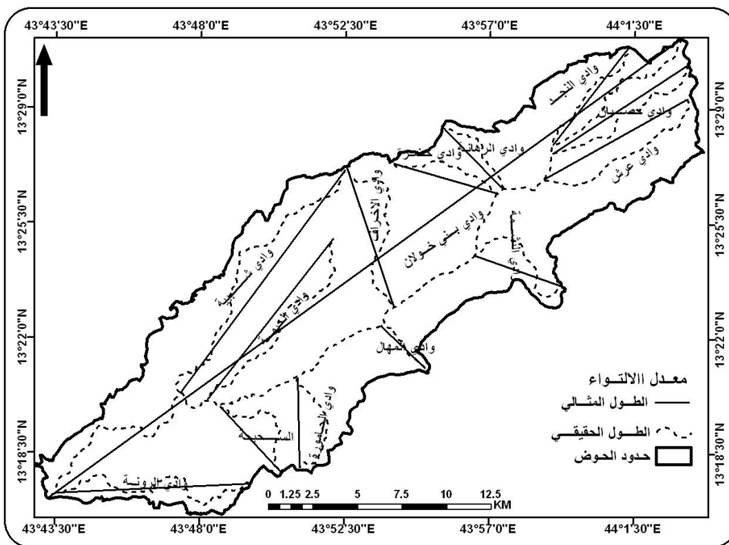
شكل (7) معدل الالتواء
