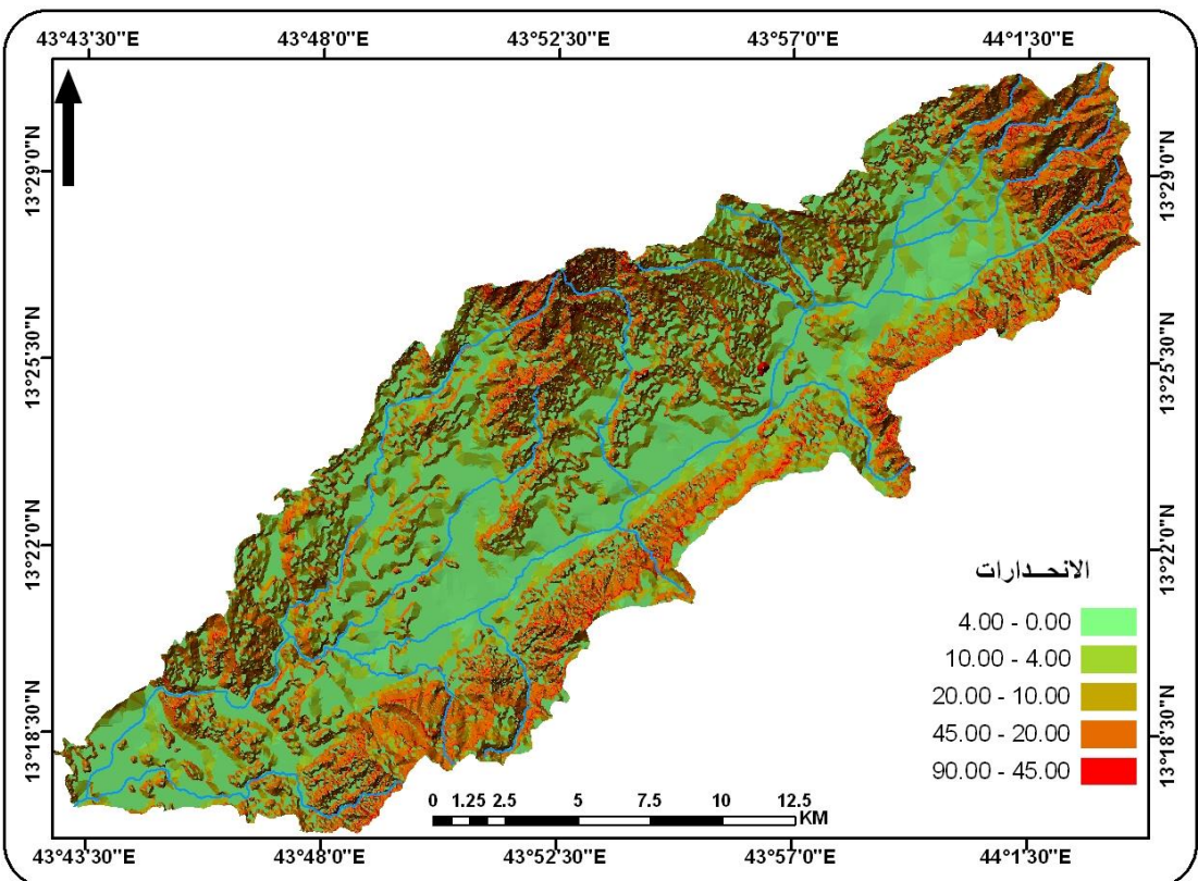
شكل (5) انحدارات الحوض
