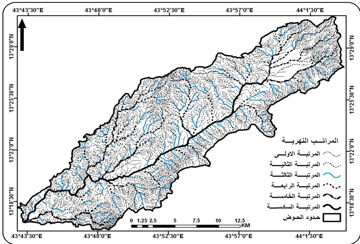
شكل (6) المراتب النهرية للحوض
