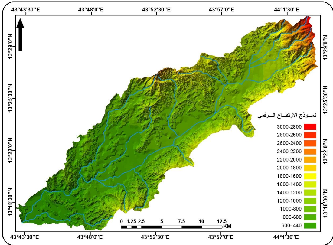
شكل (4) نموذج الارتفاع الرقمي Digital Elevation Model
