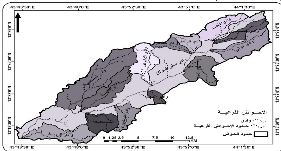
شكل (3) الأحواض الفرعية
